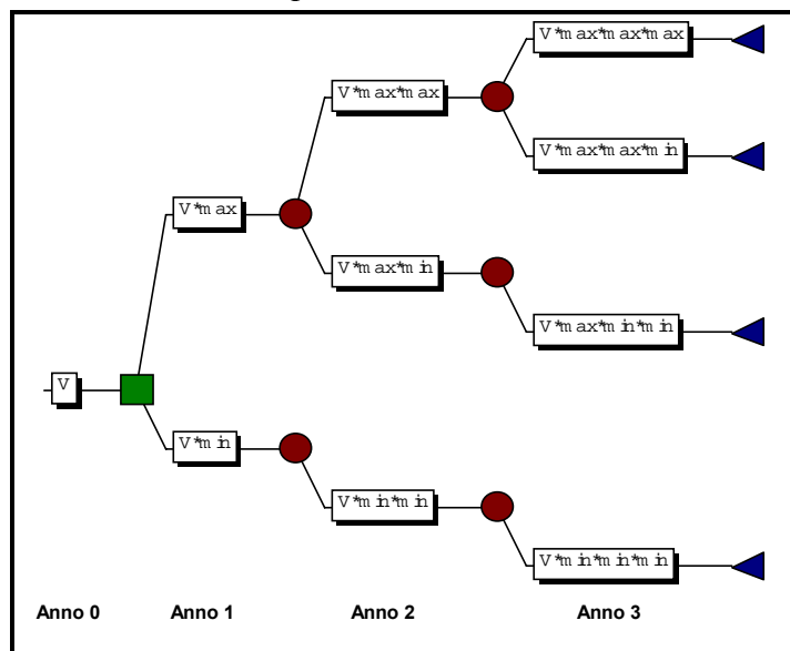
Figura 2. Processo moltiplicativo binomiale
