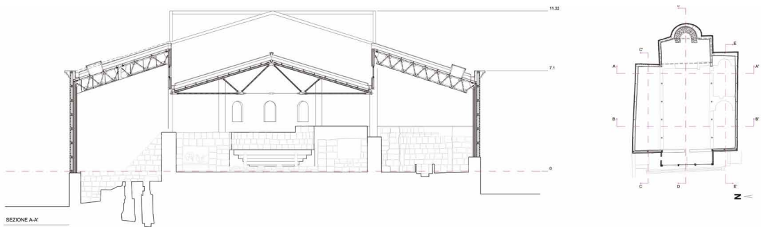
SEZIONE A-A'
